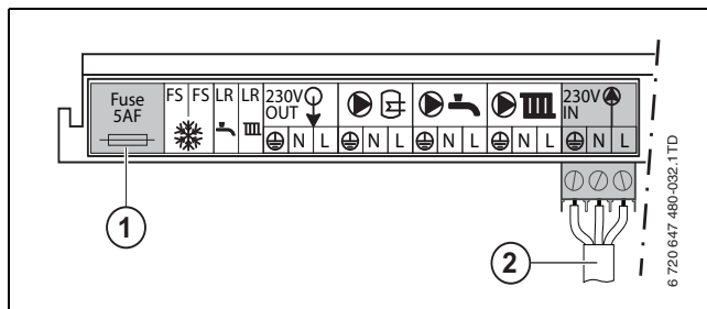
Afb. 20 Netspanningsaansluitingen
