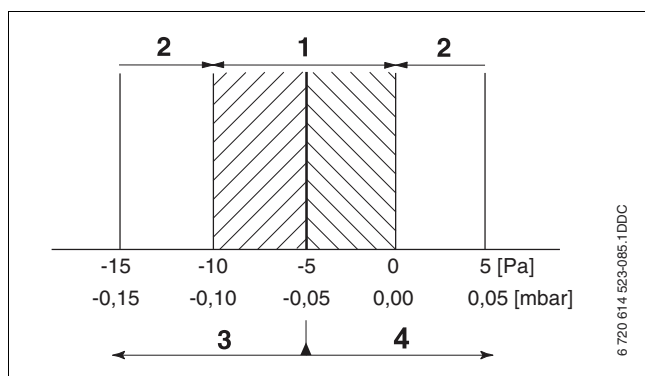
Afb. 46 Instellen drukverschil
