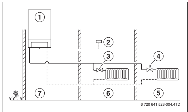
Afb. 15 Regelprincipe ruimteregeling
