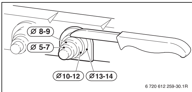
Afb. 18 Diameters kabeldoorvoeren
