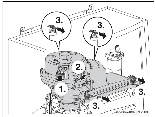
Afb. 34 Demonteren branderdekseel met ventilator
