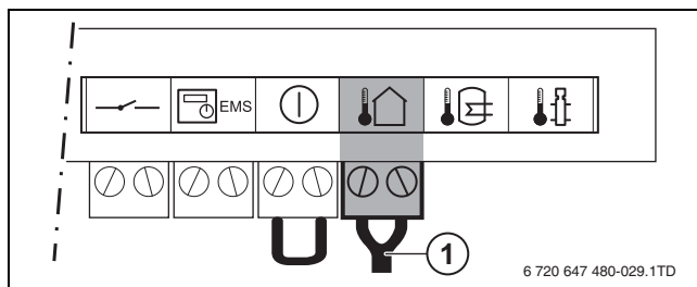
Afb. 24 Aansluiten buitentemperatuursensor
