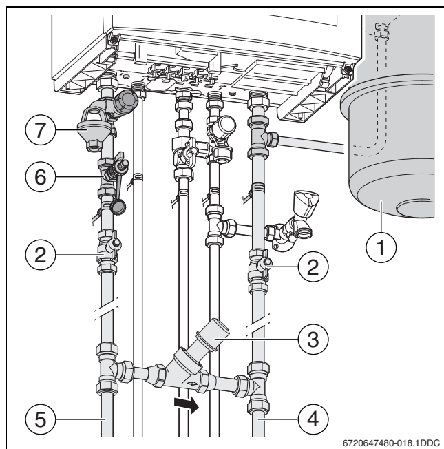
Afb. 11 Aansluiten cv-leidingen
