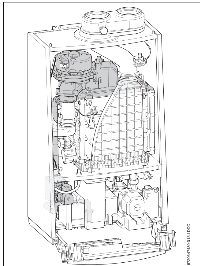
Afb. 42 Gasstraat
