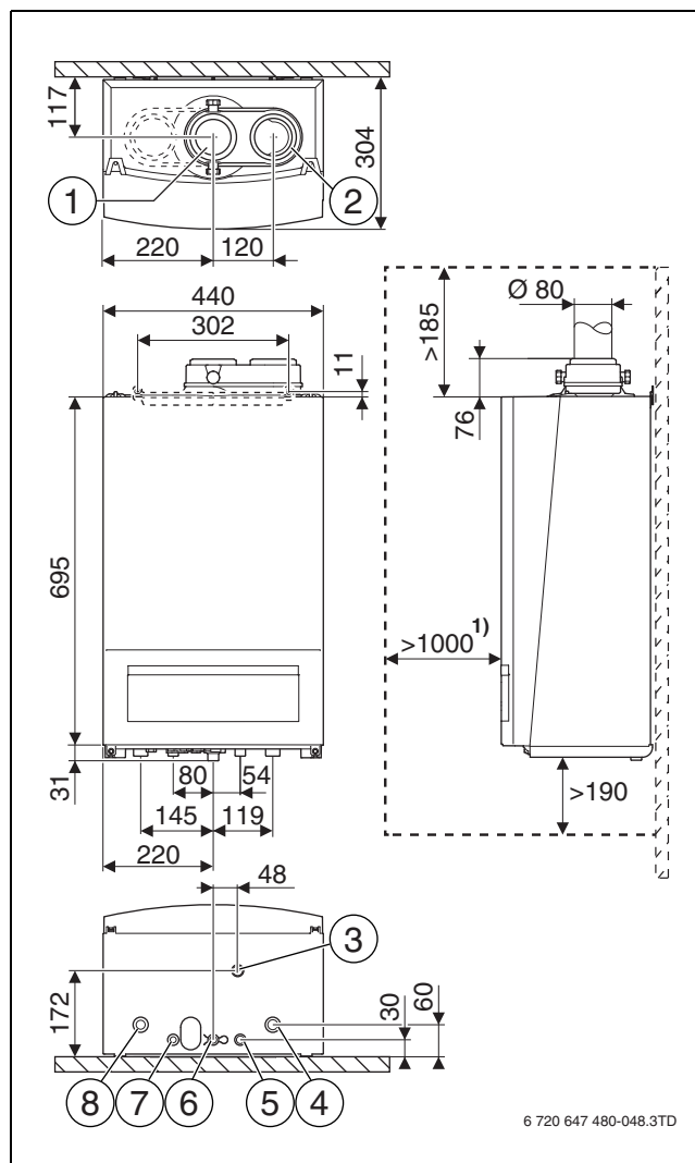
Afb. 5 Afmetingen [mm]
