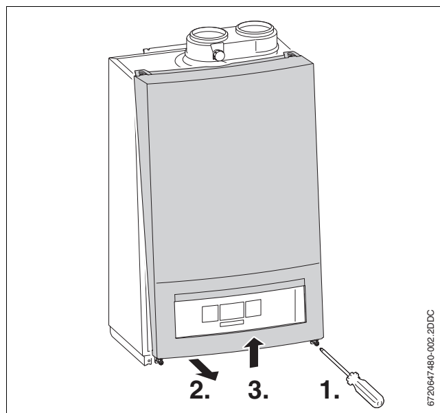
Afb. 31 Demonteren mantel
