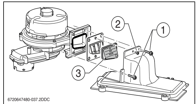
Afb. 35 Vervangen keerklep
