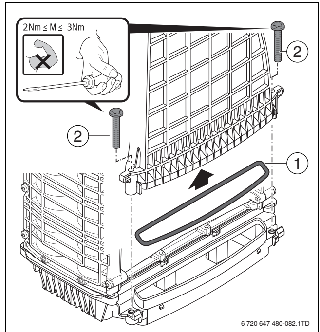
Afb. 41 Plaatsen condensbakafdichting
