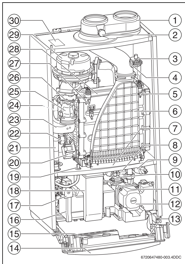
Afb. 1 Overzichtstekening
