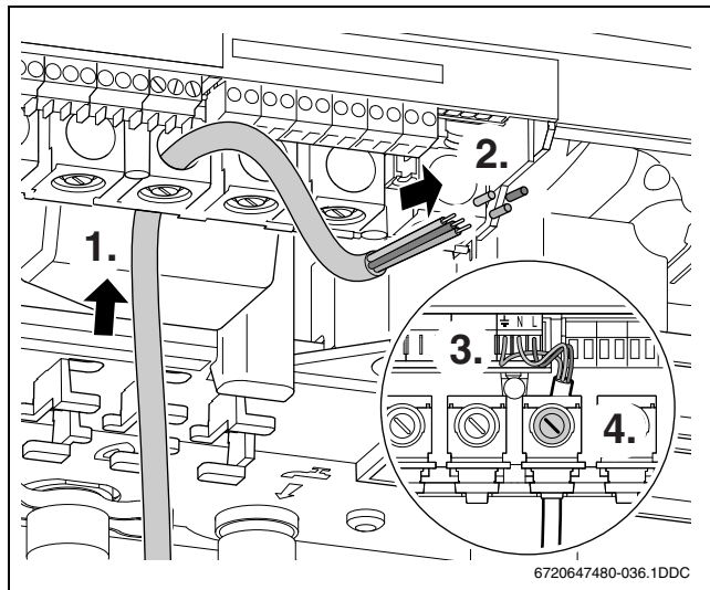
Afb. 19 Trekontlasting
