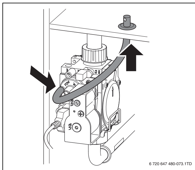
Afb. 47 Positie drukvereffeningsslang
