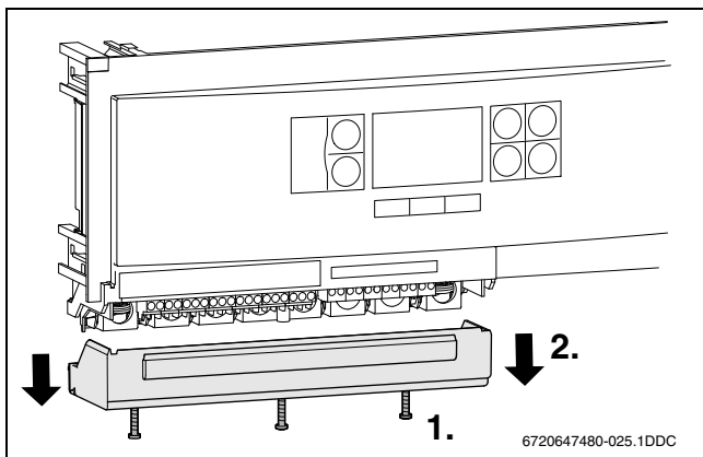
Afb. 17 Verwijderen beschermkap
