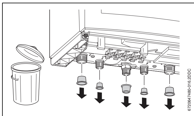
Afb. 8 Verwijderen beschermdoppen
