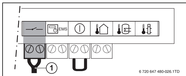
Afb. 21 Aansluiten aan-uitkamerthermostaat
