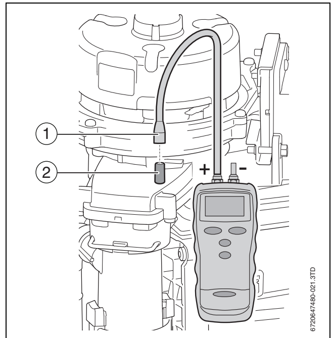
Afb. 27 Drukmeting
