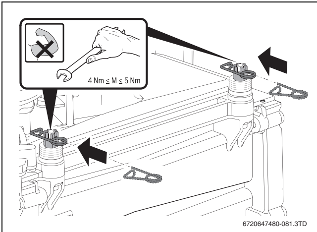
Afb. 39 Aandraaien en borgen kroonmoeren
