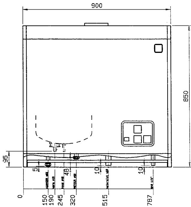
VOORAANZICHT
