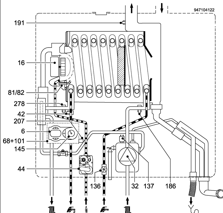
Figuur 14.6 Weergegeven type BlueSense (3-4-5) 22
