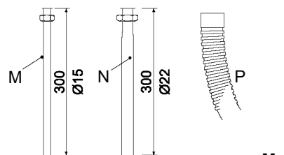
Figuur 10.1 Afmetingen en aansluitingen
