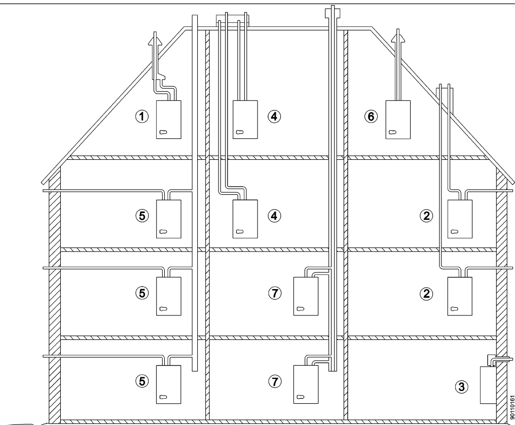
Figuur 9.4 Opstellingsmogelijkheden
