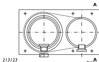
Figuur 1.2.1.2 Rookgasafvoer aansluitplaat concentrisch
