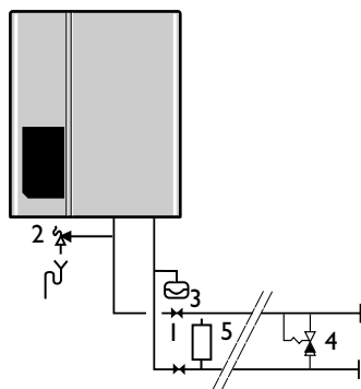
Figuur 1.3.1.3 Principeschema van Nefit EcomLine HR Single met drukverschilregelaar op afstand
