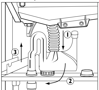
Figuur 3.2.4 Demonteren sifon
