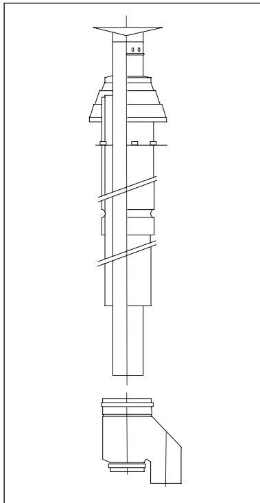
Figuur 1.2.6.2 Nefit dakdoorvoerset
