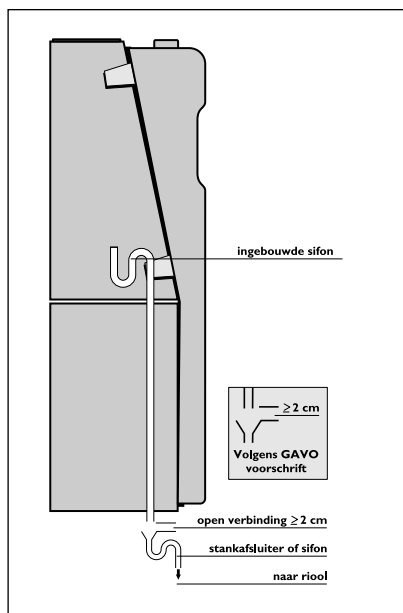
Figuur 1.2.4.1 Aansluiting condensafvoer
