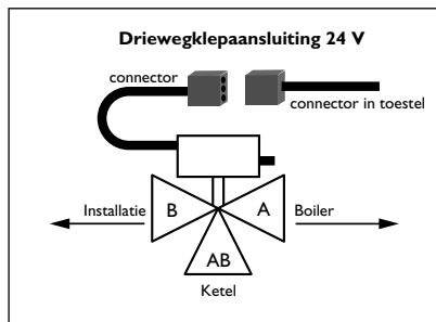
Figuur 1.3.5.1 Aansluiting driewegklep
