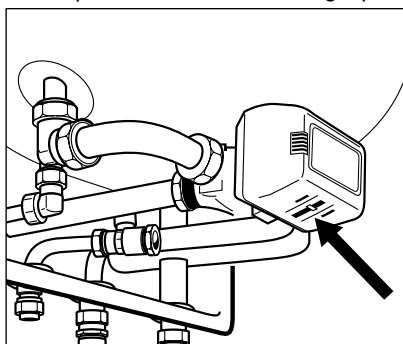
Figuur 2.1.3 Middenpositiehandel van de driewegklep
