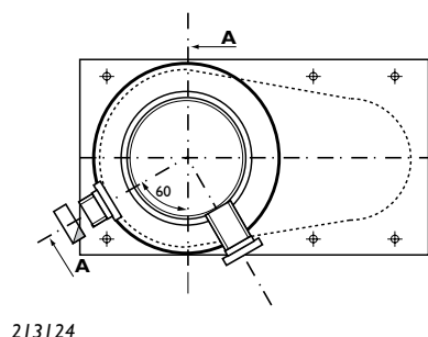
Figuur 1.2.1.2 Rookgasafvoer aansluitplaat concentrisch
