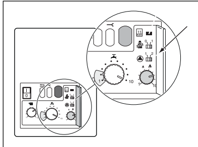
Figuur 1.3.4.1 Pompschakelaar
