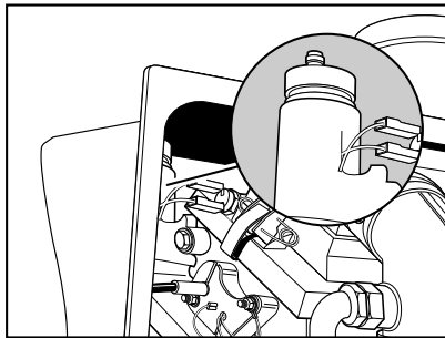
Figuur 1.3.1.1 Automatische ontlufter
