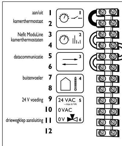
Figuur 1.4.2.1 UBA-kroonsteen
