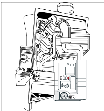
Figuur 2.3.4.2 Meten ionisatiestroom
