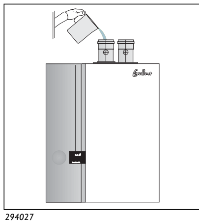
Figuur 2.2.1 Vullen sifon via rookgasafvoeraansluiting
