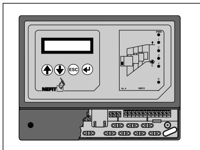
Figuur 1.4.4.1 Modulerende cascaderregelaar
