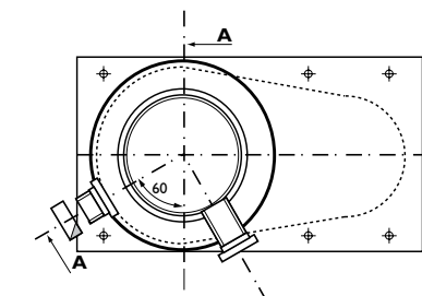
Figuur 1.2.1.2 Rookgasafvoer aansluitplaat concentrisch
