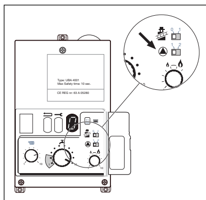
Figuur 1.3.4.1 Pompschakelaar
