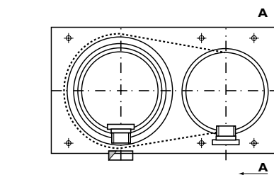
Figuur 1.2.1.1 Rookgasafvoer aansluitplaat dubbelpijps
