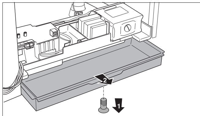
Fig. 39 Schuiflade openen
