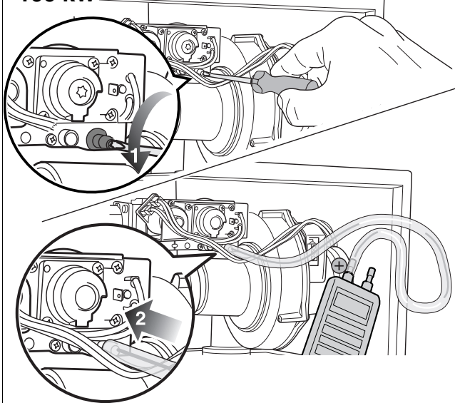
Fig. 92 Gas/lucht-verhouding controleren
