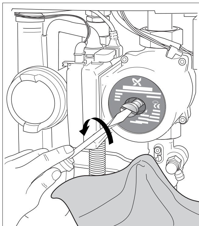
Fig. 62 Pomp ontluchten
