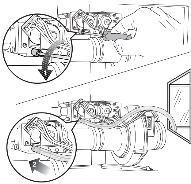
Fig. 67 Gastoevoerleiding ontluichten
